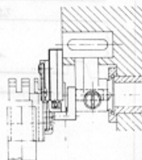
SCHEMA DI MONTAGGIO APPARECCHIATURA 136-80 CON AZIONATORE A BOTTONE DI MANOVELLA LAYOUT FOR MOUNTING THE 136-80 DEVICE WITH STARTER AND CRANK PIN
