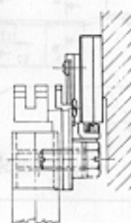
SCHEMA DI MONTAGGIO APPAR. 135-80; 136-80; 137-80 CON AZIONATORE A LEVA PER MACCHINE CON TRASPORTO DIFFERENZIALE LAYOUT FOR MOUNTING THE 135-80; 136-80; 137-80 DEVICES WITH LEVER STARTER FOR HEAD WITH DIFFERENTIAL FEED
