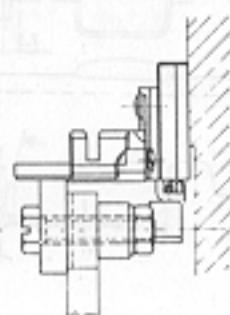
SCHEMA DI MONTAGGIO APPAR. 135-80; 136-80; 137-80 CON AZIONATORE A LEVA PER MACCHINE SENZA TRASPORTO DIFFERENZIALE LAYOUT FOR MOUNTING THE 135-80; 136-80 137-80 DEVICES WITH LEVER STARTER FOR HEADS WITHOUT DIFFERENTIAL FEED
