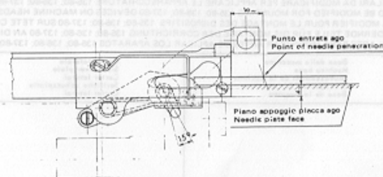
SCHEMA DI MONTAGGIO APPARECCHIATURA 136-80 CON AZIONATORE A BOTTONE DI MANOVELLA LAYOUT FOR MOUNTING THE 136-80 DEVICE WITH STARTER AND CRANK PIN
