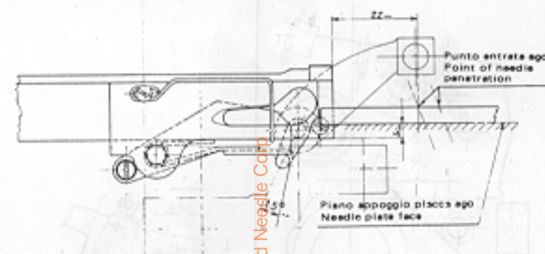
SCHEMA DI MONTAGGIO APPAR. 135-80; 136-80; 137-80 CON AZIONATORE A LEVA PER MACCHINE CON TRASPORTO DIFFERENZIALE LAYOUT FOR MOUNTING THE 135-80; 136-80; 137-80 DEVICES WITH LEVER STARTER FOR HEAD WITH DIFFERENTIAL FEED
