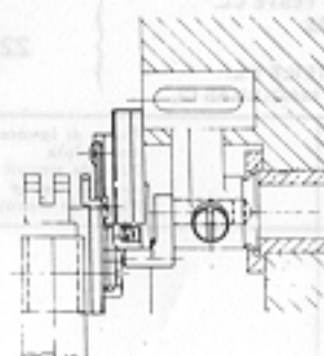
SCHEMA DI MONTAGGIO APPARECCHIATURE 135-80 e 137-80 CON AZIONATORE A BOTTONE DI MANOVELLA LAYOUT FOR MOUNTING THE 135-80; 137-80 DEVICES WITH STARTER AND CRANK PIN
