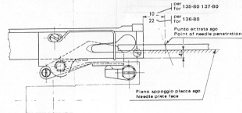
SCHEMA DI MONTAGGIO APPAR. 135-80; 136-80; 137-80 CON AZIONATORE A LEVA PER MACCHINE SENZA TRASPORTO DIFFERENZIALE LAYOUT FOR MOUNTING THE 135-80; 136-80 137-80 DEVICES WITH LEVER STARTER FOR HEADS WITHOUT DIFFERENTIAL FEED
